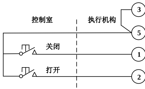
图 9-2 保持式打开/关闭控制，行程可逆，但不能停在中途位置
