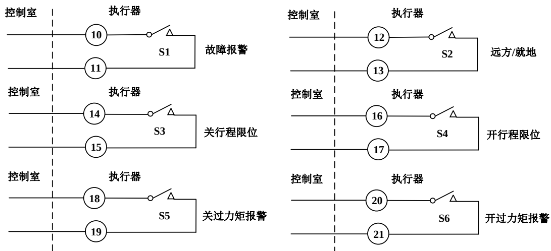
图 9-6 S1~S6 输出触点接线图
