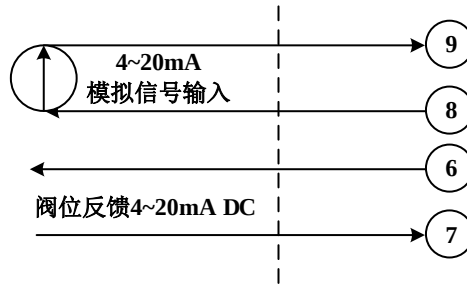
图 9-5 远程模拟量控制线路图
