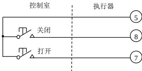
图 8-1 点动式打开/关闭控制，执行器可以停在中途任意位置
